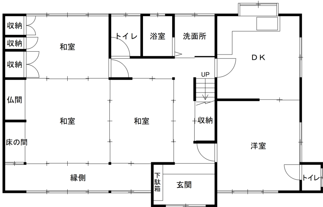
1階平面図
